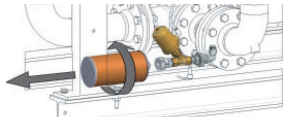
Schalldämpfer lösen
