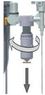
Steuerluftfilter öffnen
