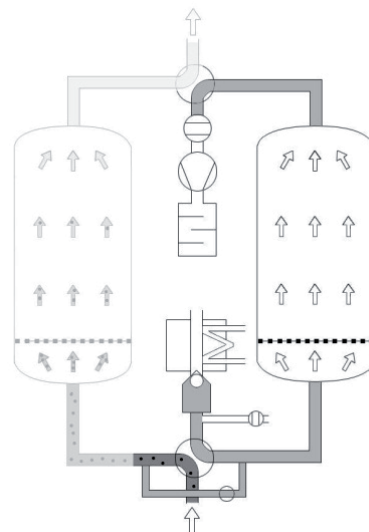
Druckaufbau
