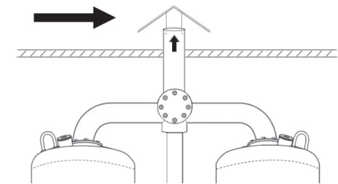
Wetterschutz bei Verlegung der Leitung nach oben
