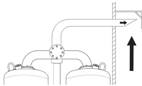
Wetterschutz bei seitlicher Verlegung der Leitung
